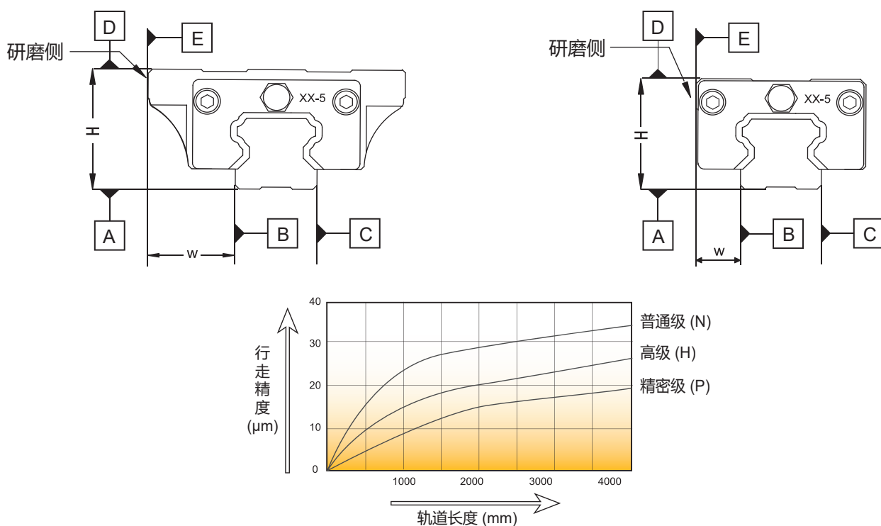
图1.6.1 ABBA直线导轨的行走精度
